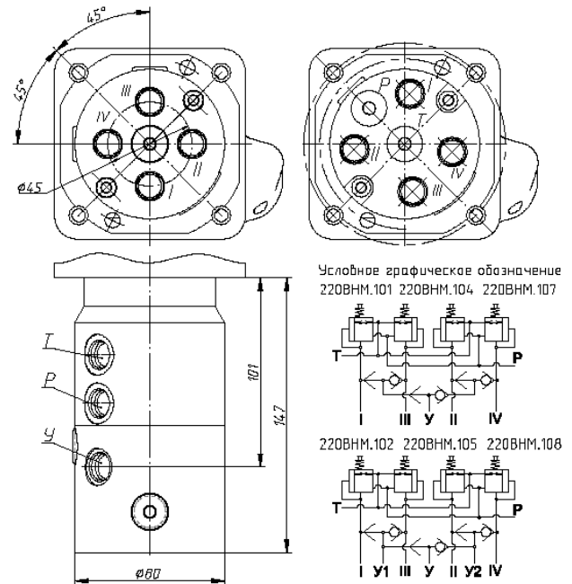
Рисунок 1 - Блоки управления четырехзолотниковые с одной рукояткой серии 220ВНМ.100, варианты рукояток
