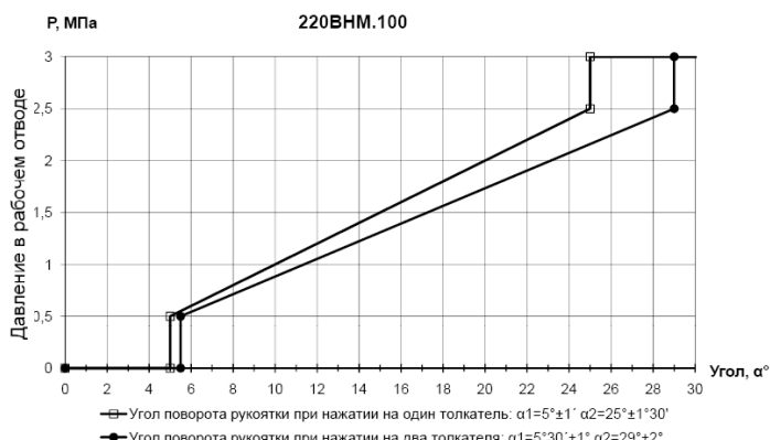
Рисунок 4 – Зависимость редуцированного давления от угла поворота
